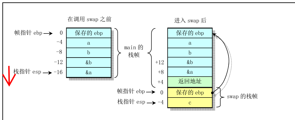
图 3-5 调用函数 main 和 swap 的栈帧结构
