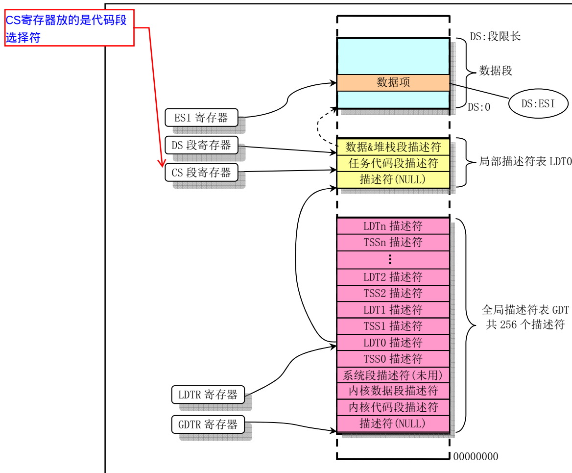
图 6-12 Linux 内核使用描述符表的示意图。
